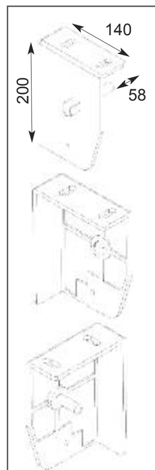
supporti in alluminio estruso
