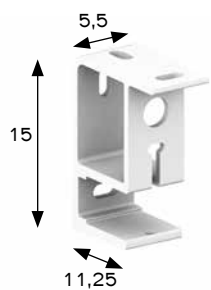
PIASTRA A PARETE/SOFFITTO ① (di serie)
