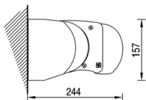
INSTALLAZIONE A PARETE 0° - 75°
