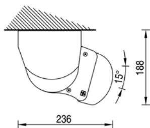
INSTALLAZIONE A SOFFITTO 15° - 90°
