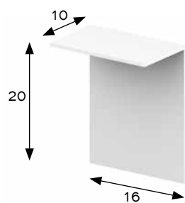
PIASTRA ATTACCO A SPALLINA SPIGOLI AL VIVO (fornita senza fori)
