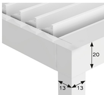
PARTICOLARE ANGOLO
